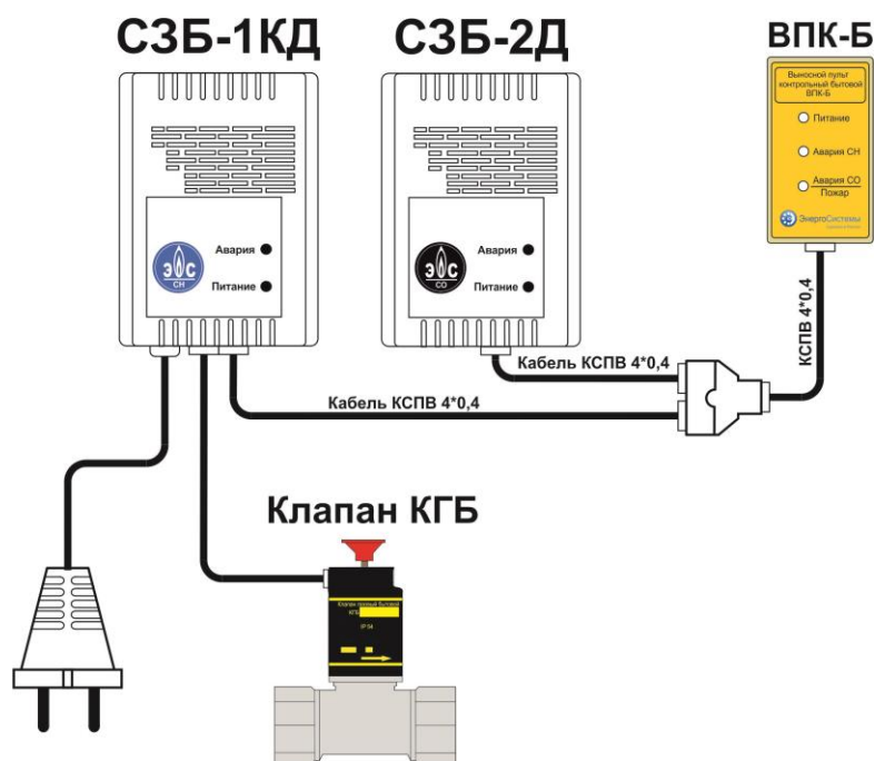
Рис.В.1 – Общий вид системы СКЗ «Кристалл – 2 – мини» с подключением пульта контрольного ВПК-Б.
