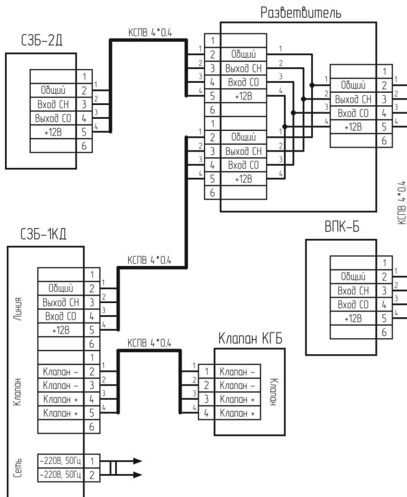
Рис.В.1 – Общий вид системы СКЗ «Кристалл – 2 – мини» с подключением пульта контрольного ВПК-Б.
