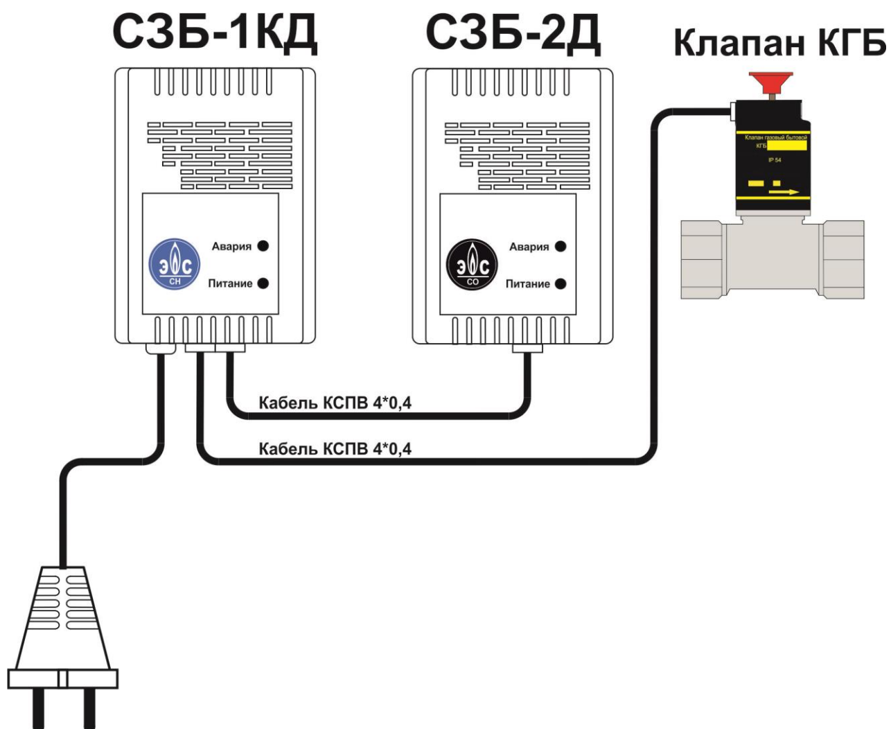
Рис.А.1 СКЗ «Кристалл-2- мини», стандартная комплектация
