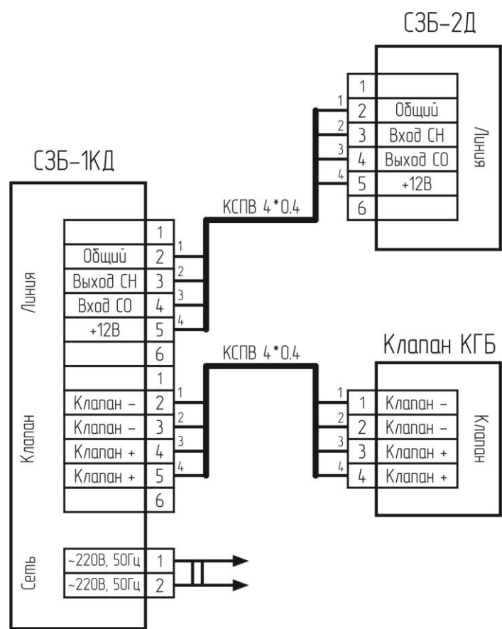
Рис. Б.1. Схема подключения электрическая.
